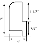
CHICAGO Z-FRAME CZF
