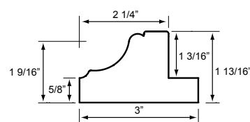
Deco Frame DFO
