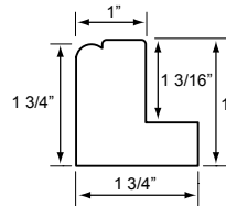
DECO SILL FRAME DSO
